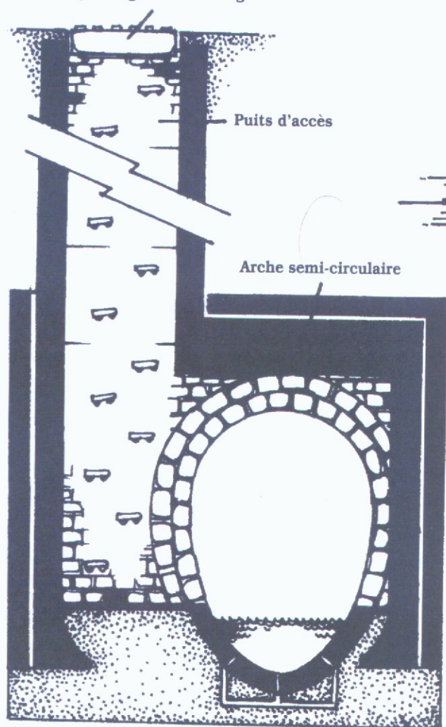
Vue transversale
