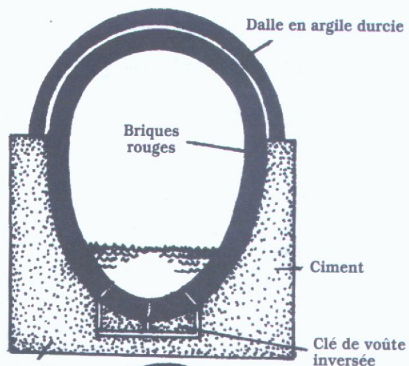
Vue transversale
